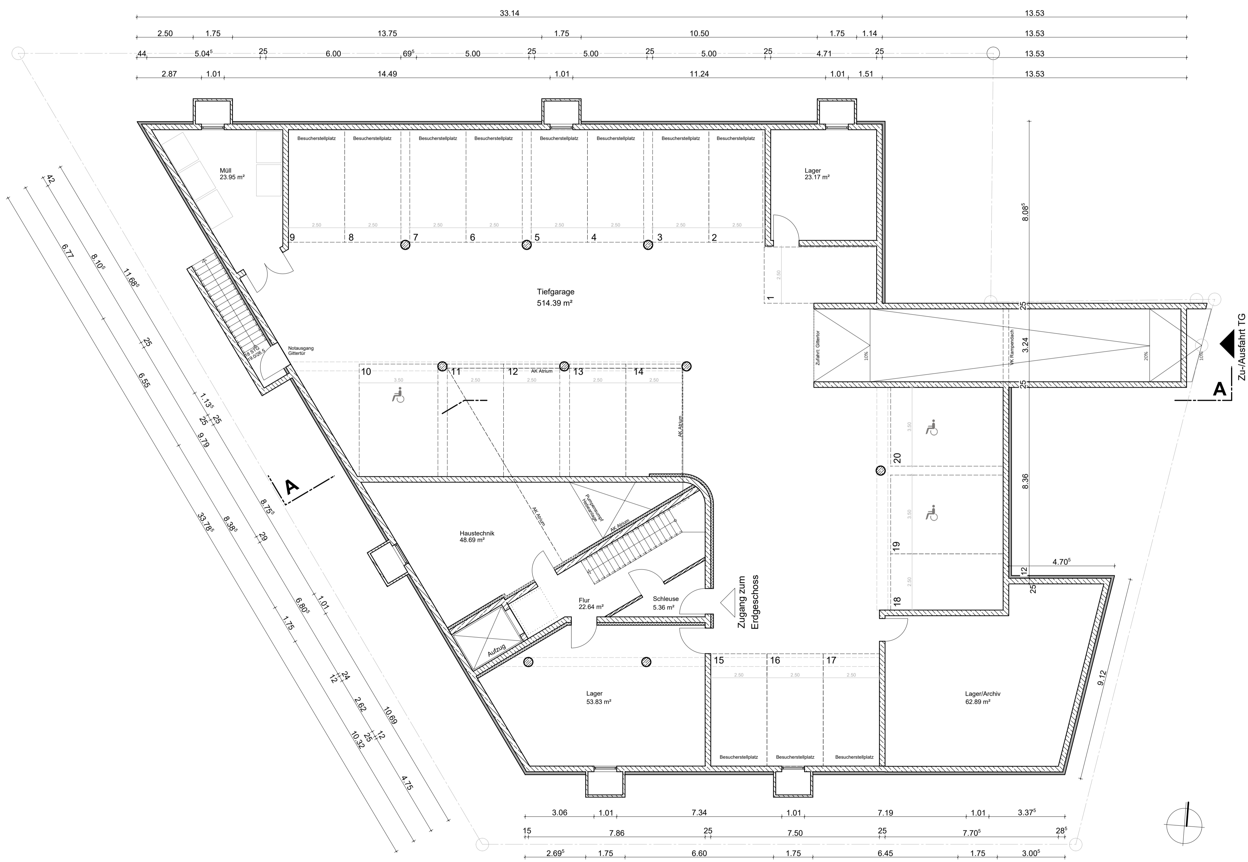
UNTERGESCHOSS
