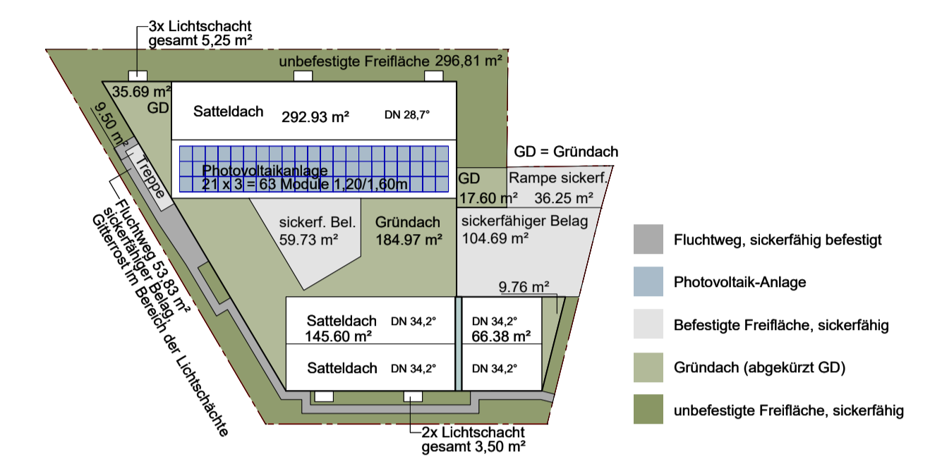
DACHAUFSICHT / BEFESTIGTE FLÄCHEN 1:500
